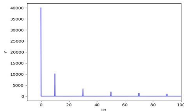
放大器饱和输出信号频谱图
