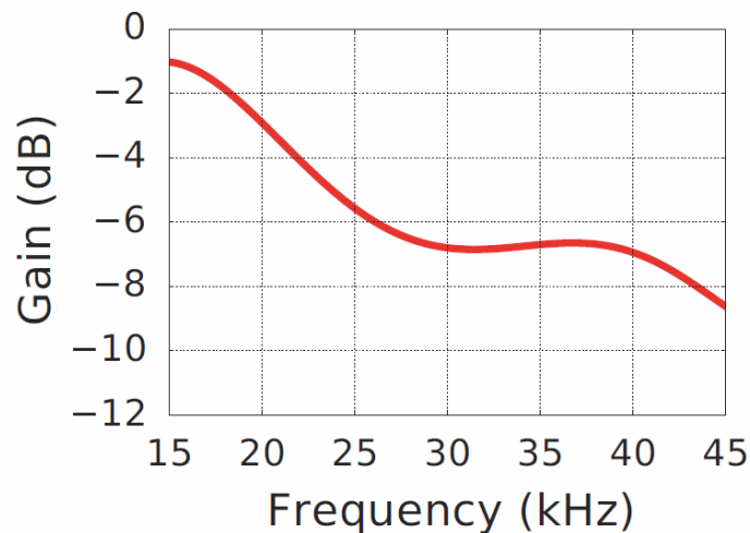
麦克风频率响应 (>15kHz)
