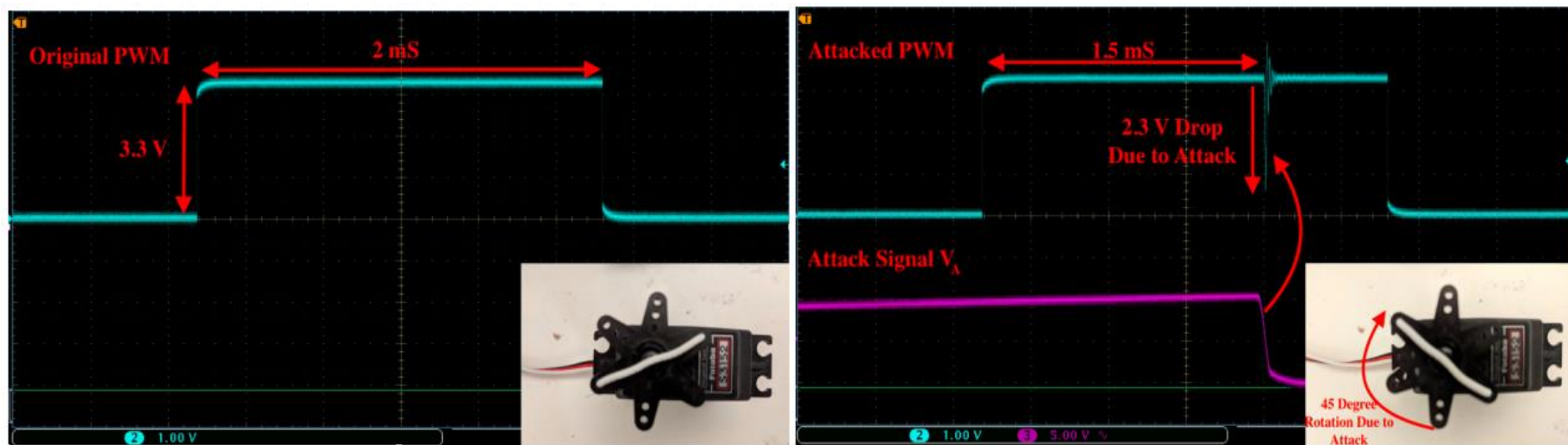
(b) 攻击信号 V_A （紫色）；被攻击PWM信号（蓝色）和对应的伺服电机位置
