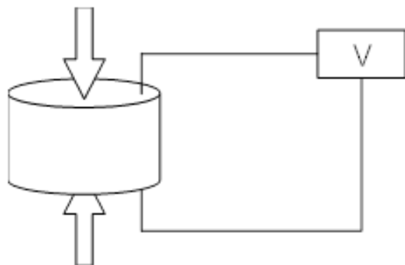
压电效应
